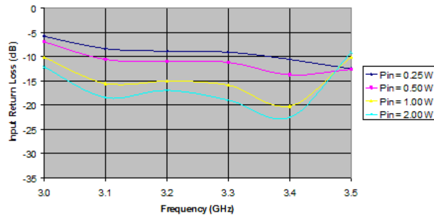
ILT3035M15: 100us / 10% / 28V / I_{DQ} -10\text{mA}
