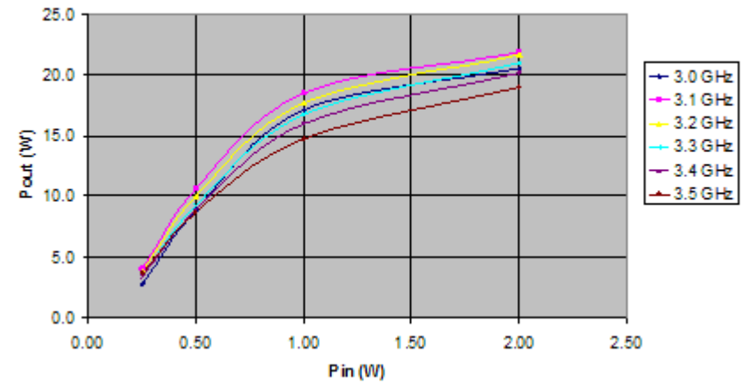
ILT3035M15: 100us / 10% / 28V / I_{DQ} -10\text{mA}
