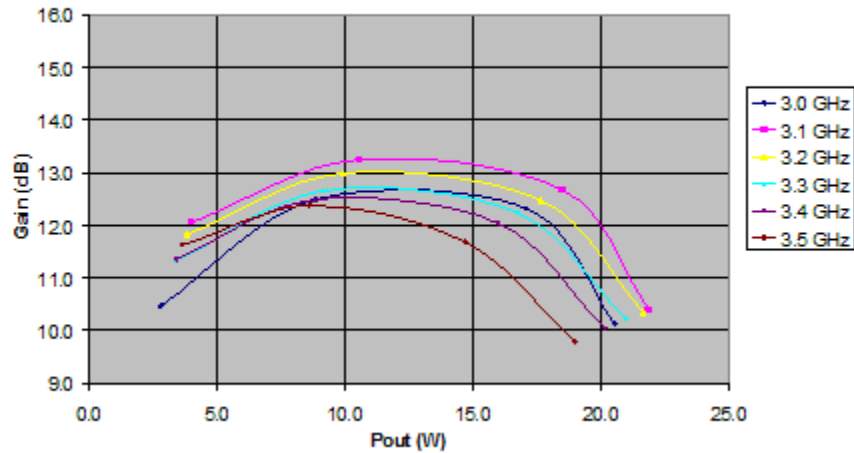
ILT3035M15: 100us / 10% / 28V / I_{DQ} -10\text{mA}
